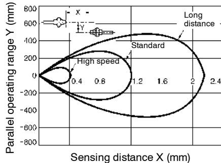
E32-T11 with E3JU-XR amplifier
