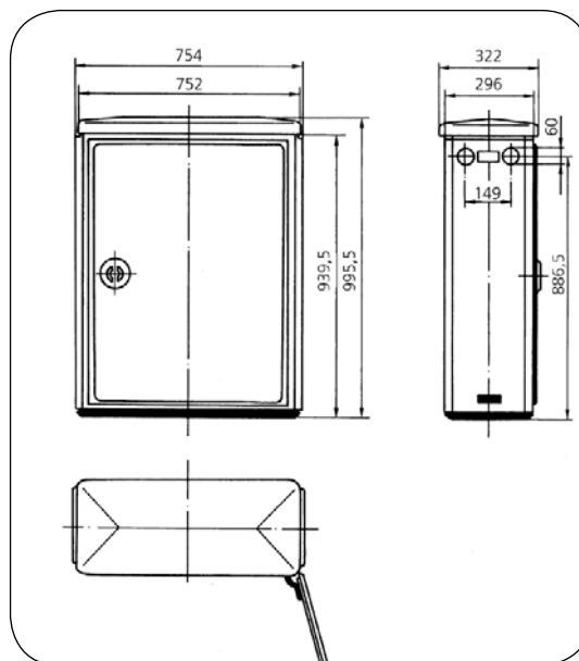
Maßbild: Kabelverzweiger 59m1
