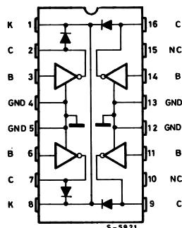
ULN2064B ULN2066B
