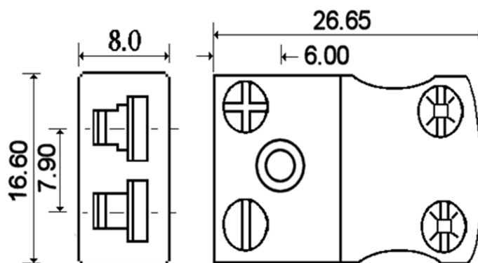
Miniature Socket
