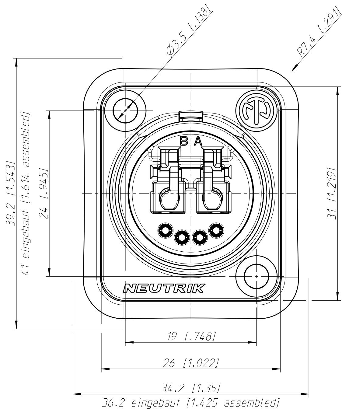
Frontplattenausschnitt Rueckseite Panel Cutout Rearside
