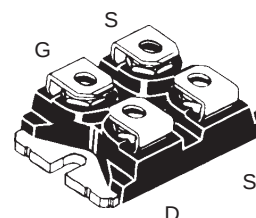
miniBLOC, SOT-227 B (IXFN) E153432
