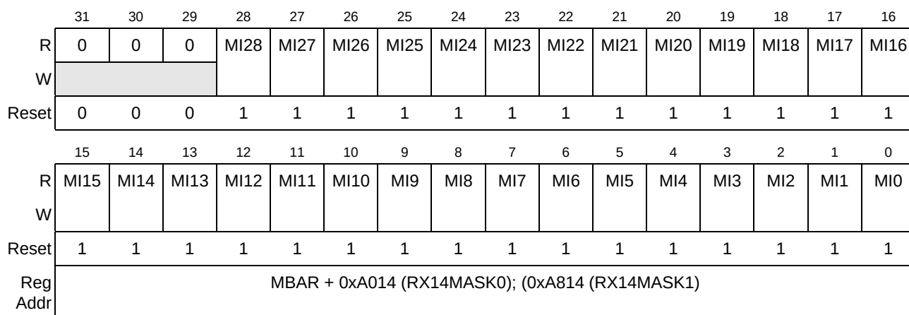
Figure 21-8. FlexCAN Rx14 Mask Register
