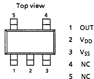
(3) SOT-23-5
