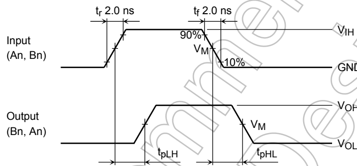
図 2 t_{pLH} , t_{pHL}
