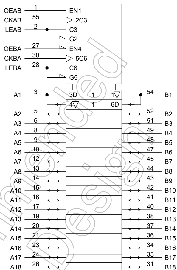
論理図
