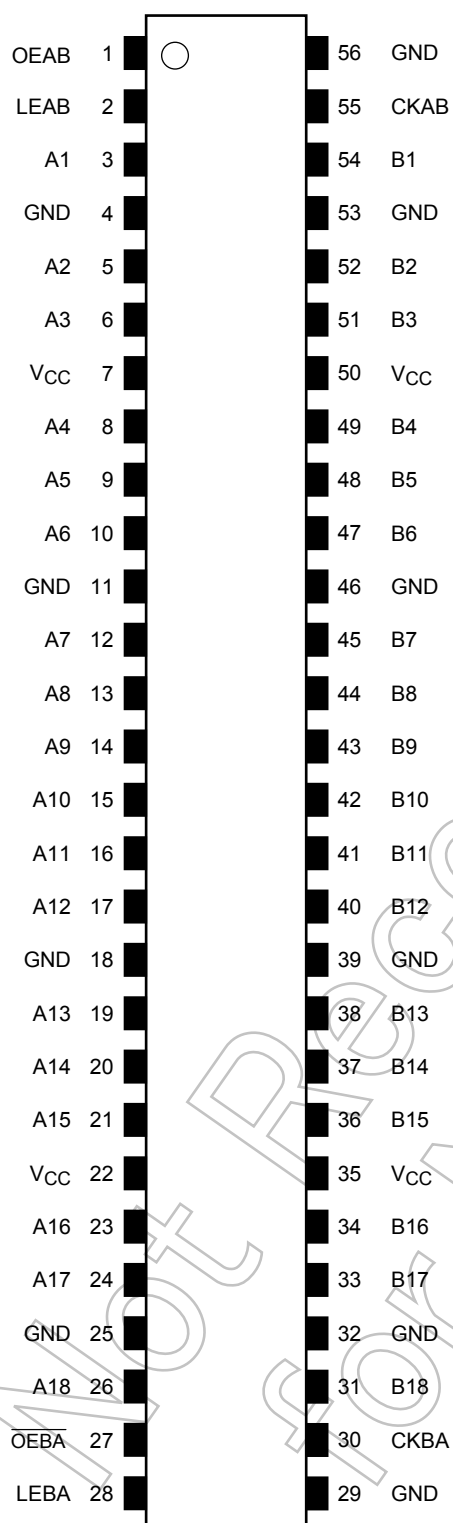
ピン接続図 (top view)
