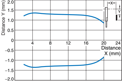
Reflective E32-L56E
