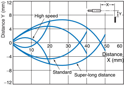
Reflective E32-D24
