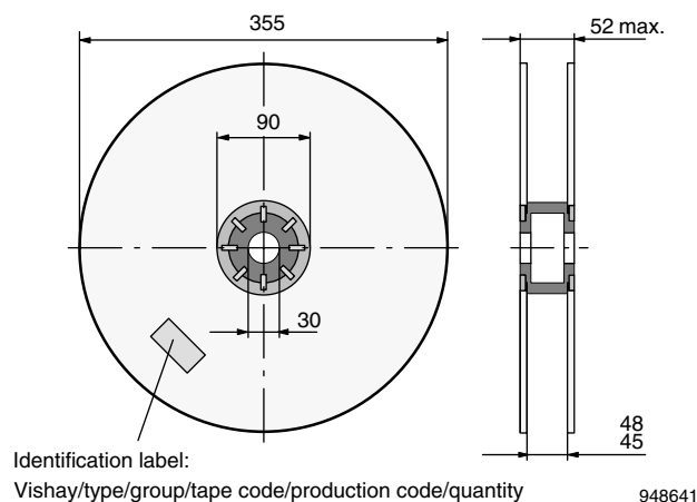
Fig. 18 - Reel Dimensions
