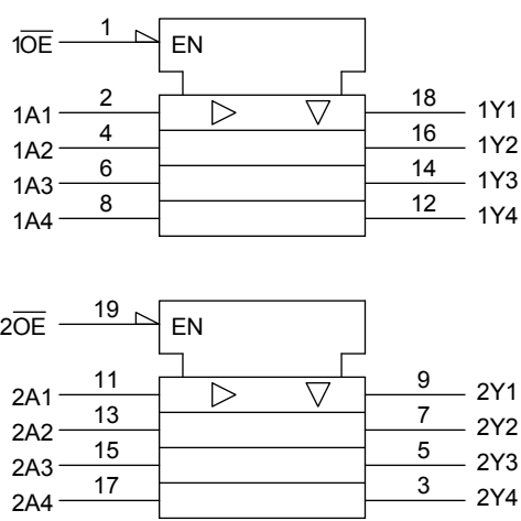
論理図
