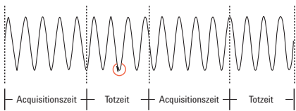
Abbildung 3. Reduzierung der Totzeit zwischen Auffrischungen ...
