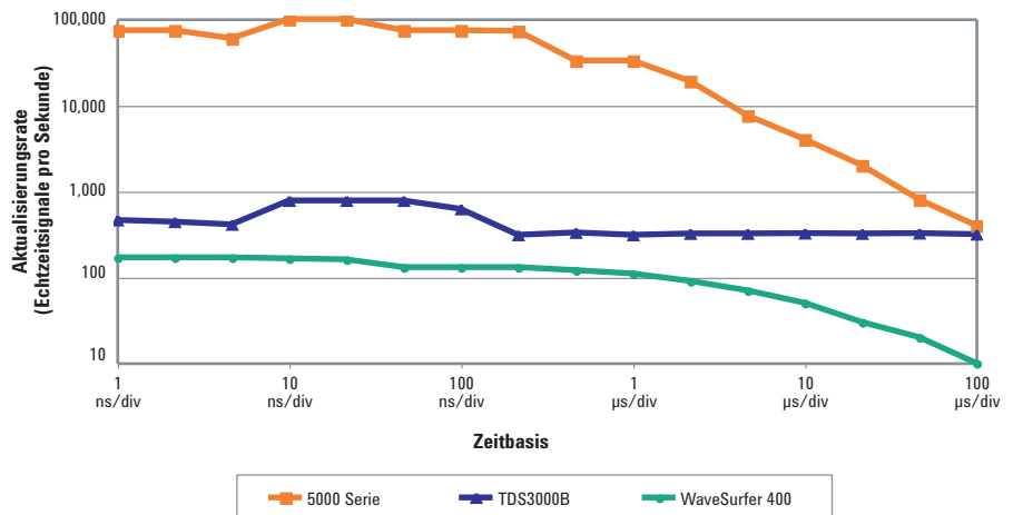
Abbildung 5. Aktualisierungsraten gängiger Oszilloskope unter Verwendung ihres standardmäßigen Zeitauffrischungsmodus in Echtzeit
