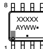
SOIC8, SOIC-8 EP
