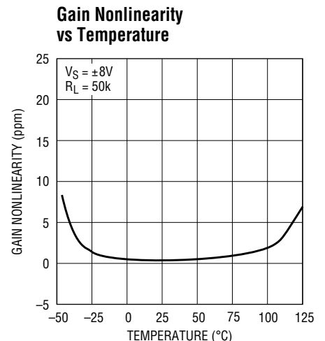
LTC1100 • TPC03
