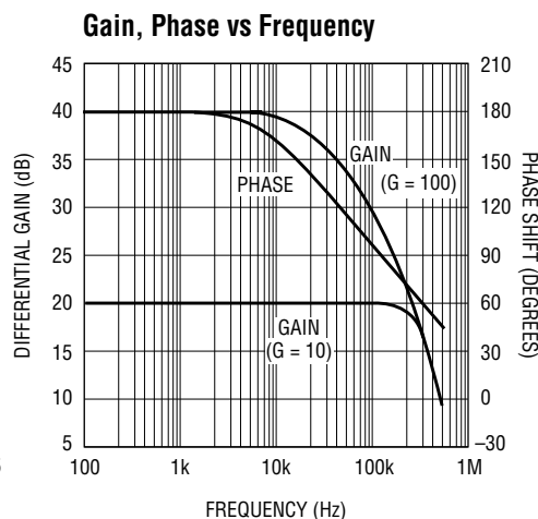
LTC1100 • TPC02
