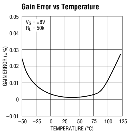
LTC1100 • TPC01
