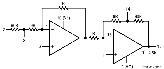
LTC1100 • BD02
