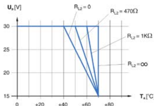
Fig. 2: Temperaturminderung / Réduction de température Temperature derating
