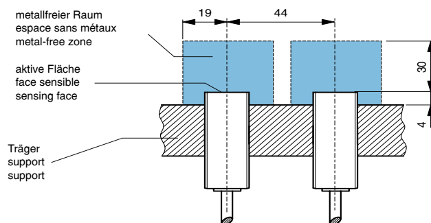
Fig. 3: Einbau / Montage / Installation
