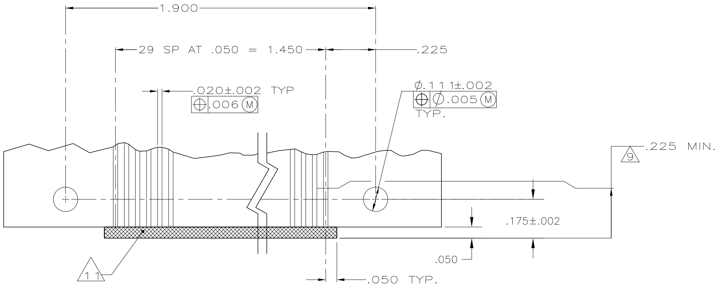
RECM. .P.C. BD. LAYOUT
