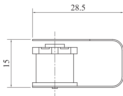
Dimensions : Millimetres
