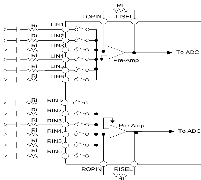
Figure 21. Input ATT
