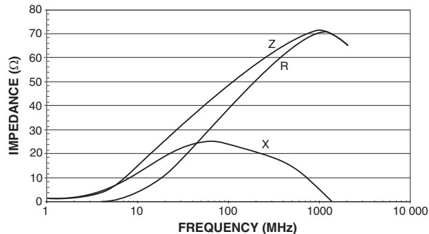
ILBB-0805 40 \Omega
