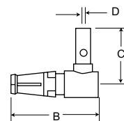
Receptacle
