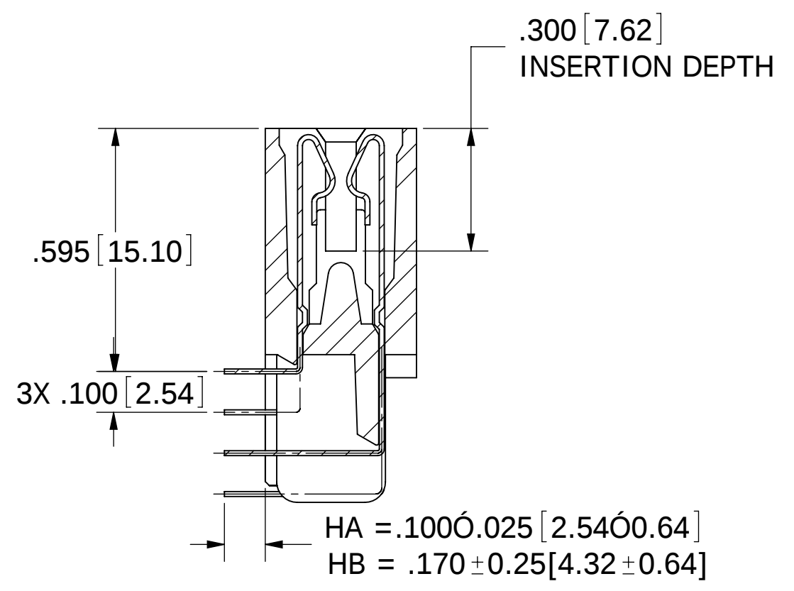
SECTION A-A SCALE 3 : 1
