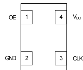
Si510 (CMOS)
