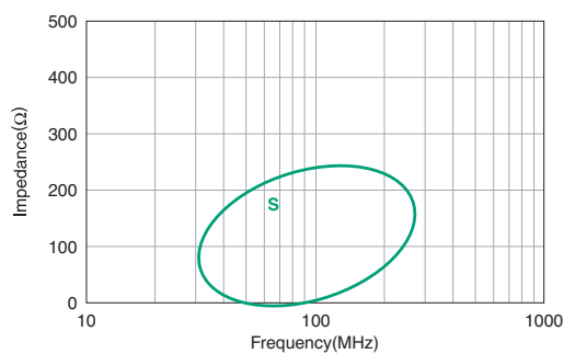
MMZ0603 Type
