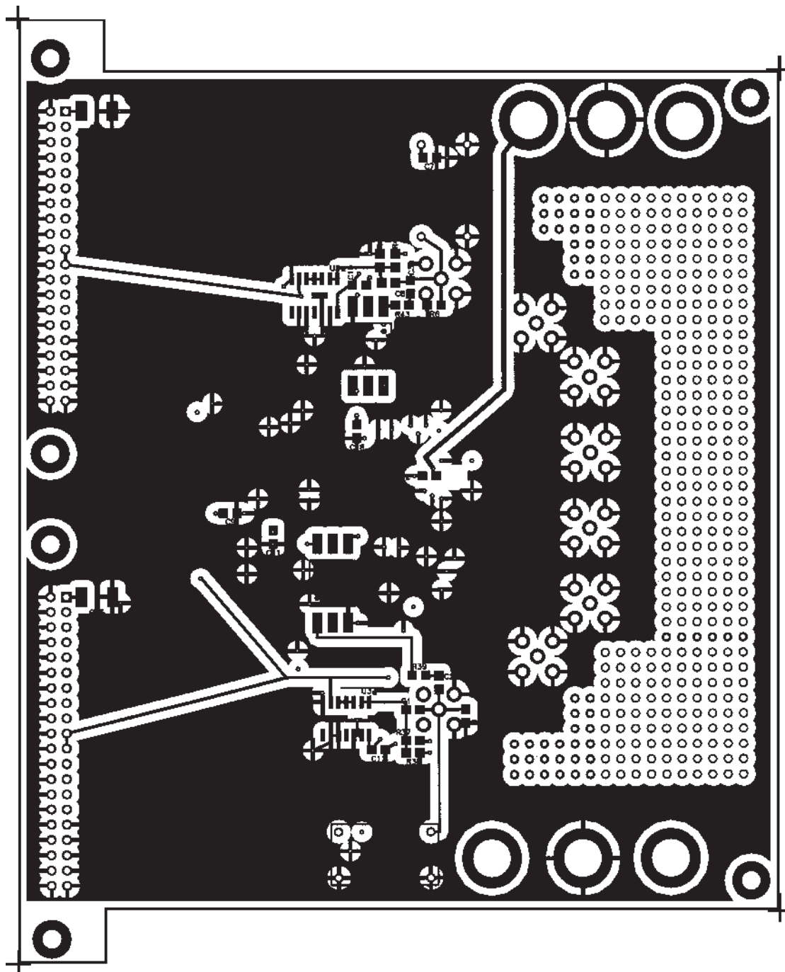
Figure 24. Bottom Layer
