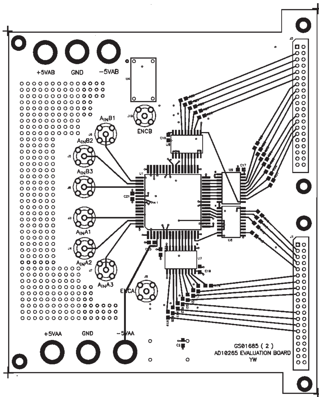
Figure 23. Top Layer
