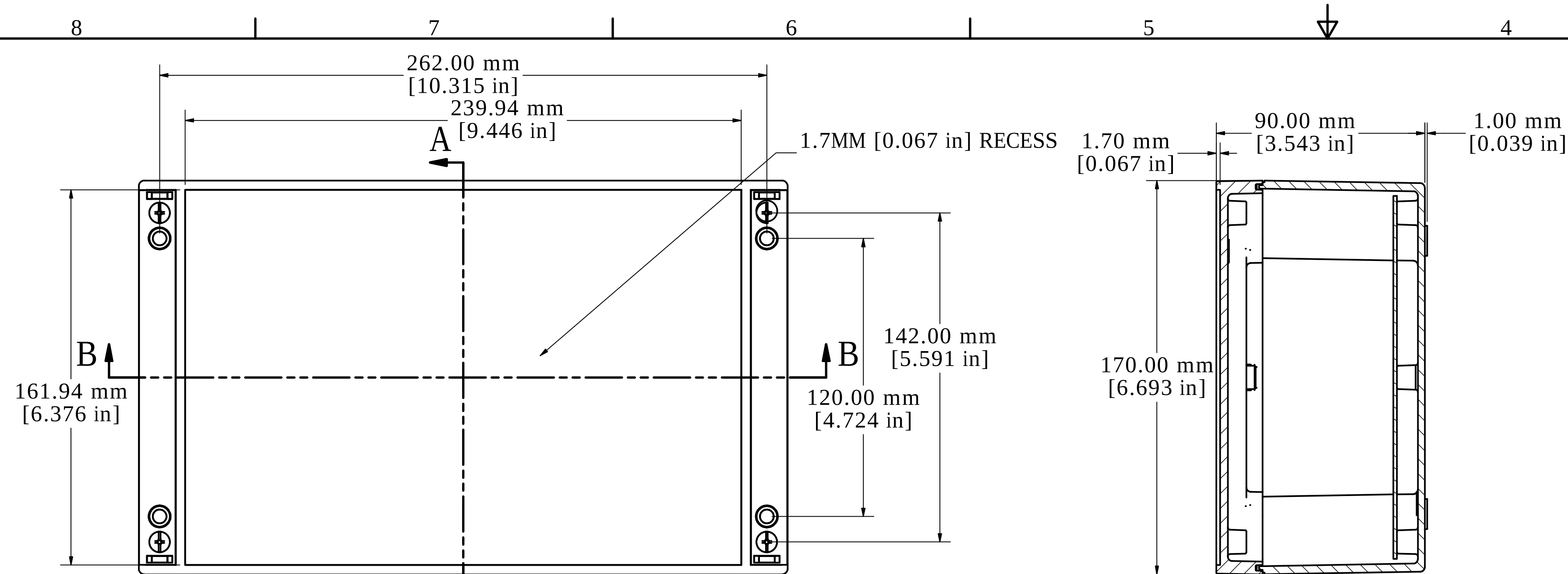
SECTION A-A
