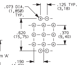
7301MD9_BE 3PDT
