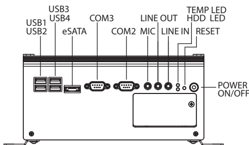
ARK-3440F
