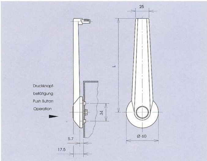
Einschließlich Schrauben DIN 84-M4 und Scheiben DIN 125. Including screws DIN 84-M4 and washers DIN 125.
