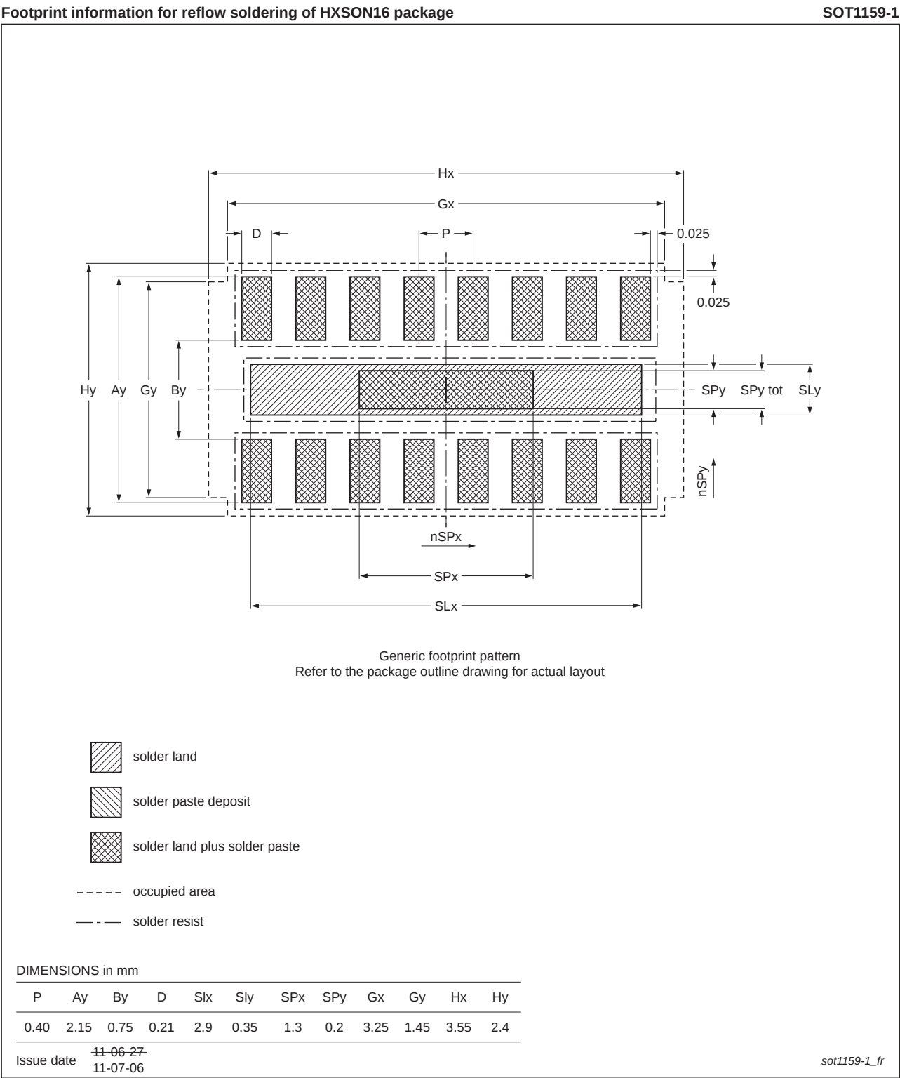
Fig 18. Reflow soldering PEMI8QFN (SOT1159-1/HXSON16)
