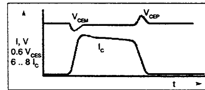
SCSOA conditions V_{CE} = 0.6 V_{CES} , V_{CEM} = 0.5 V_{CES} , V_{CEP} < V_{CES} , T_J = 125^\circ\text{C}
