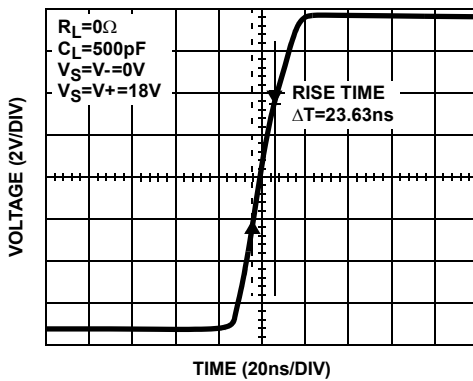
FIGURE 3. RISE TIME OUTPUT 12V p.p
