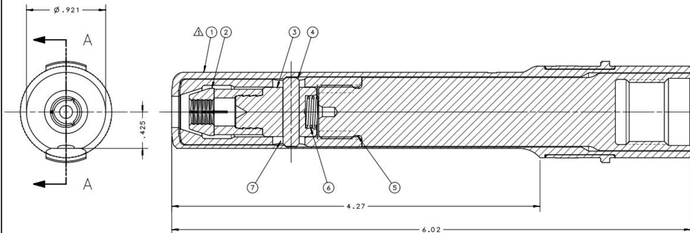
SECTION A-A
