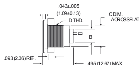
Receptacle
