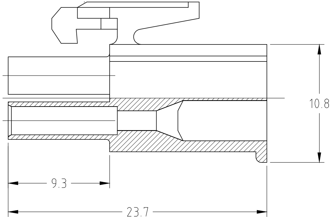
SECT A-A
