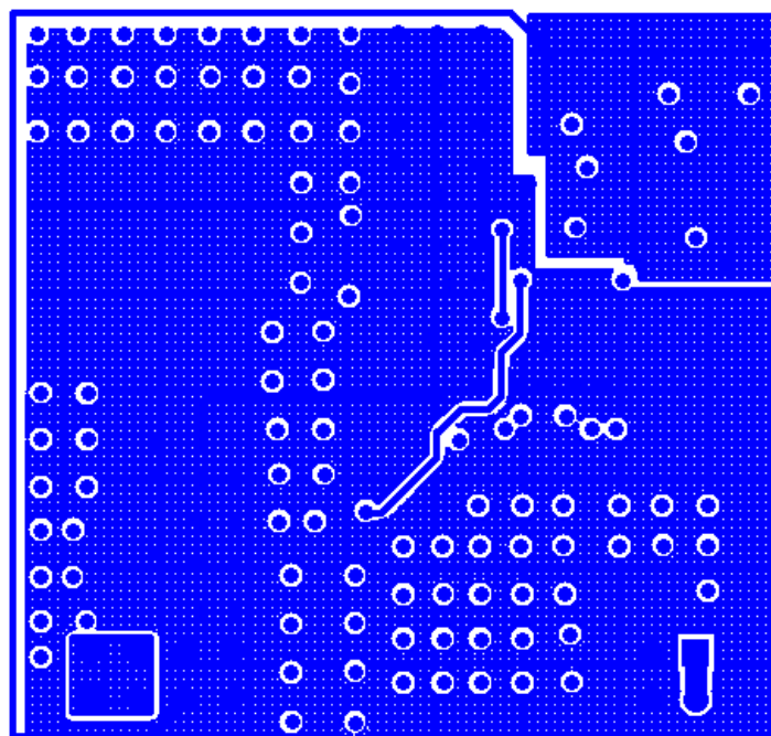
(INTER LAYER 1)
