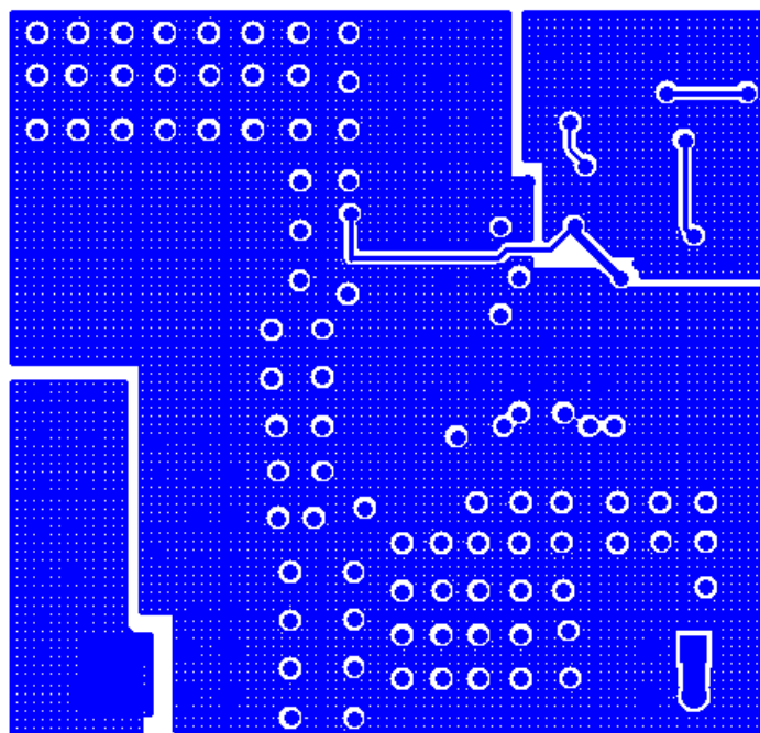
(INTER LAYER 2)
