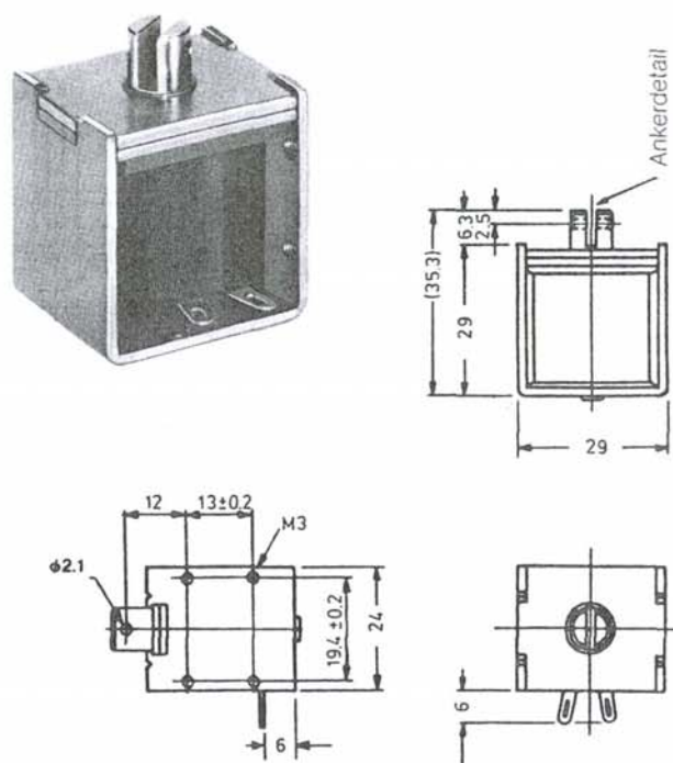
Ankerdetail
