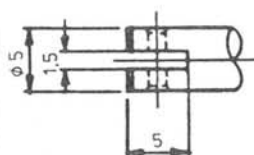
Ankerdetail
