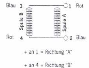
Parallelschaltung, 6 VDC
