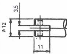
Ankerdetail
