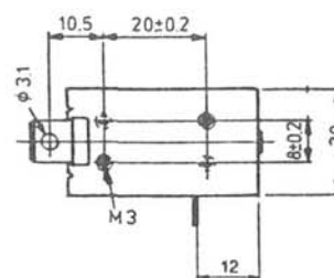
Ankerdetail
