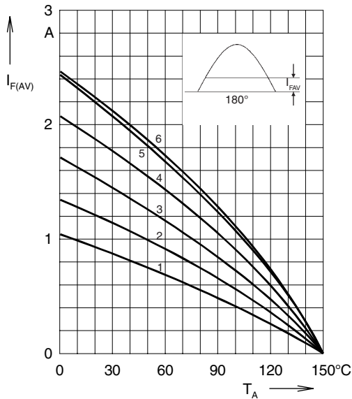
Fig. 4: Load diagramm
