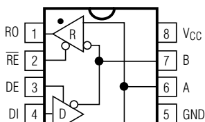
DIP/SO
