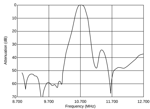
SFELF10M7GALP03-B0
