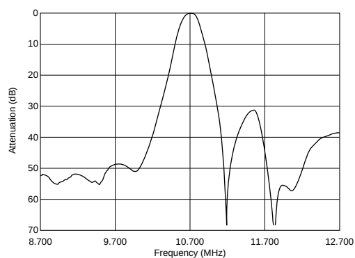
SFELF10M7GAXA-B0
