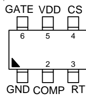
SOT-23-6
