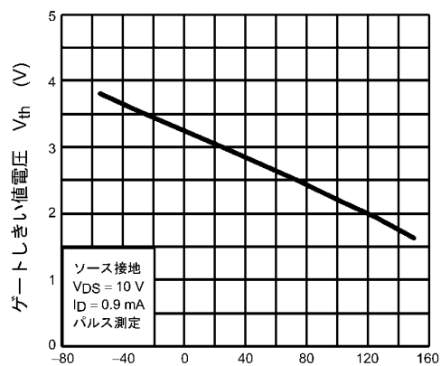
図 8.10 V th - T a
