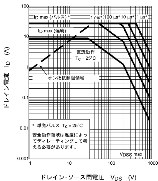
図 8.14 安全動作領域 (最大値 (保証値))
