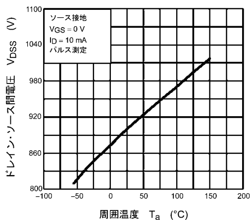
図 8.5 V_{DS} - T_a
