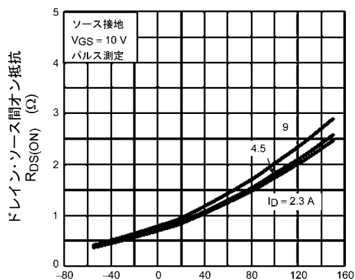
図 8.7 R DS(ON) - T a
