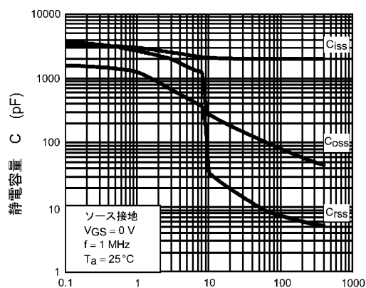
図 8.9 C - V DS
