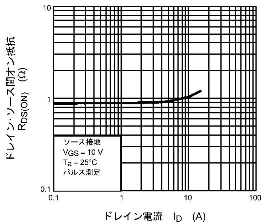
図 8.6 R_{DS(ON)} - I_D
