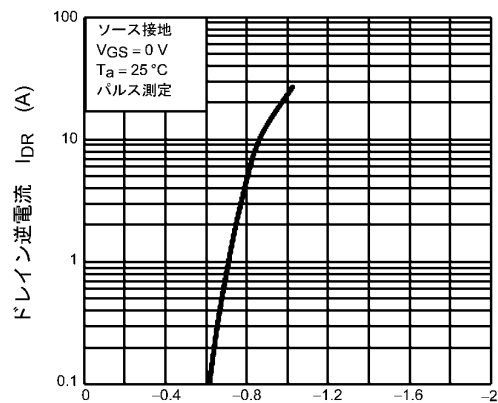
図 8.8 I DR - V DS
