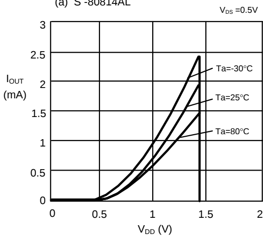
(a) S-80814AL
