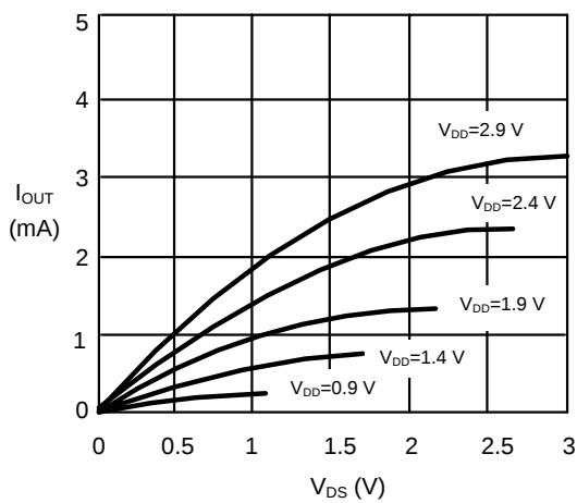
(a) S-80808AL
