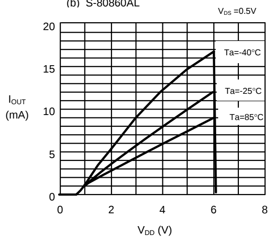
(b) S-80860AL
