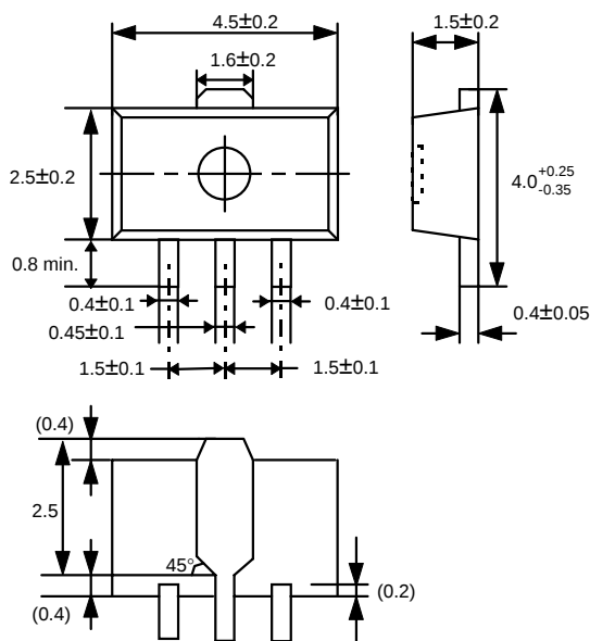
(3) SOT-89-3
