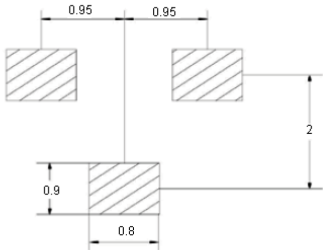
Dimensions : Millimetres
