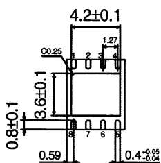
SON008V5060 (unit:mm)
