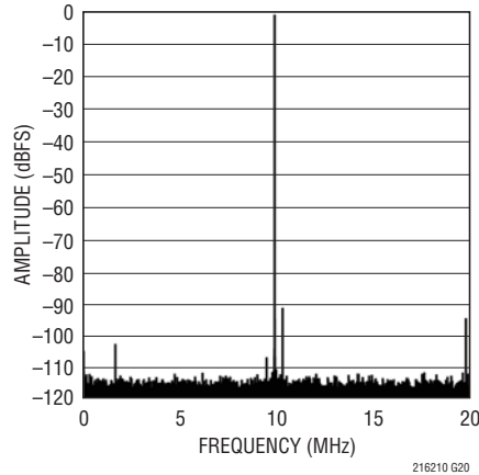
LTC2161: 64k Point FFT, f_{IN} = 70\text{MHz} , -1\text{dBFS} , 40\text{Mps}
