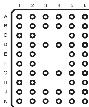
97U877AHLF 52-Ball BGA
