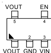
SOT-23-5
