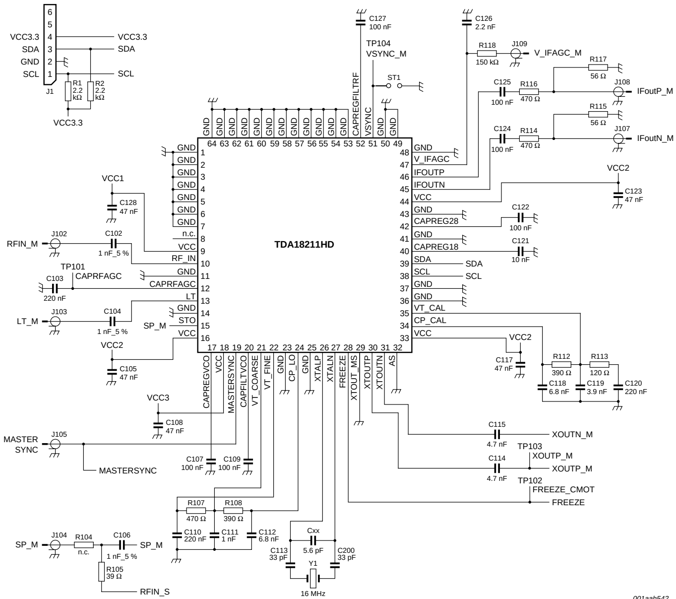
Fig 26. Test circuit
