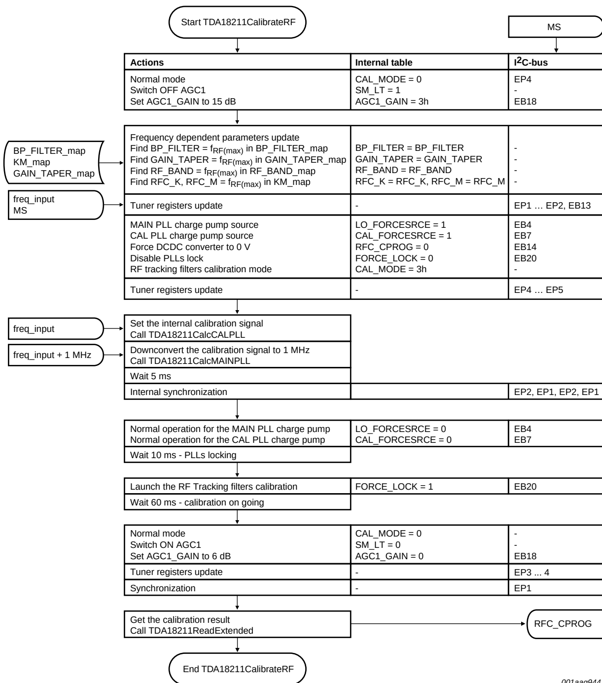
Fig 14. Flowchart TDA18211CalibrateRF
