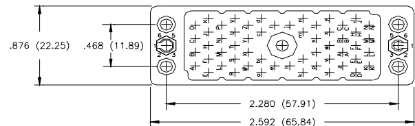
90 PIN RECEPTACLE
