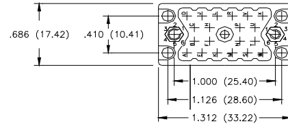
20 PIN RECEPTACLE
